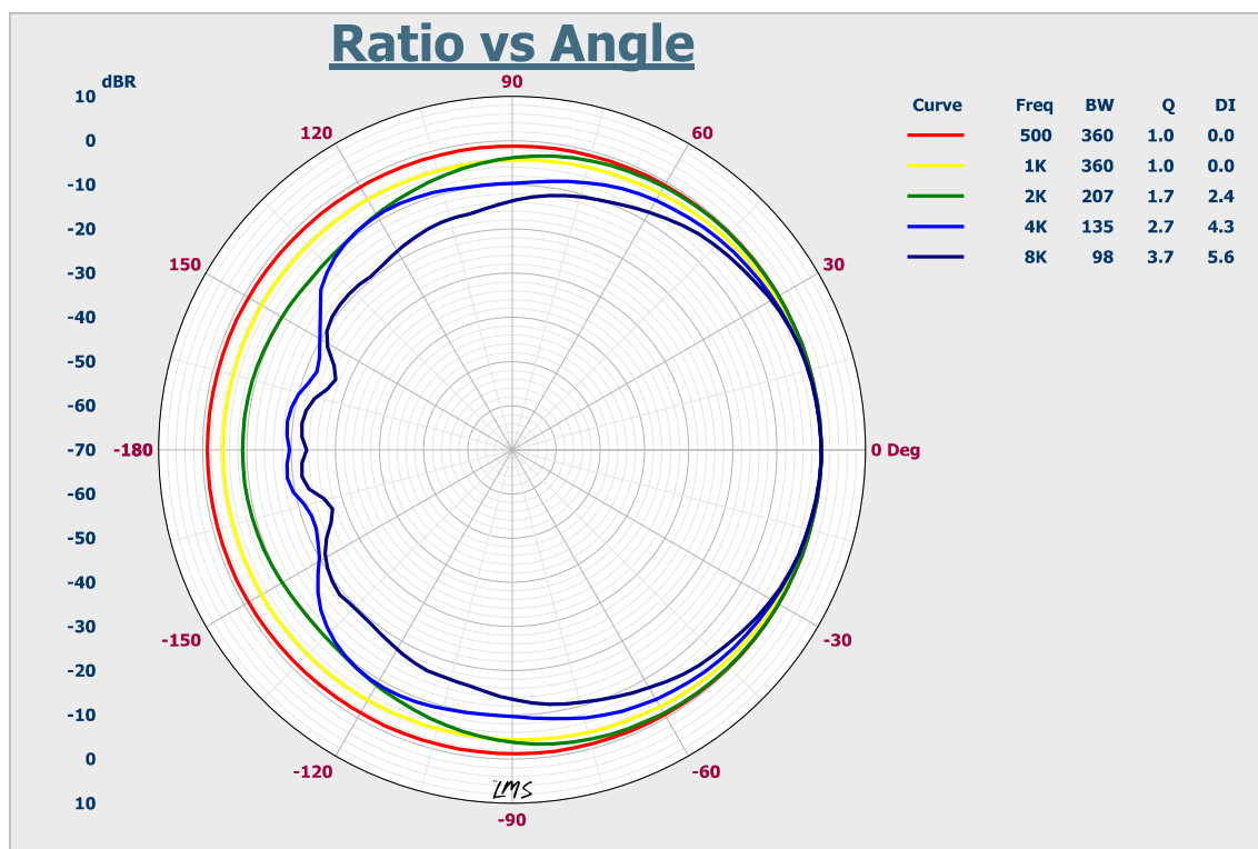
Круговая диаграмма направленности громкоговорителя LPA-40CA (цвет белый)
